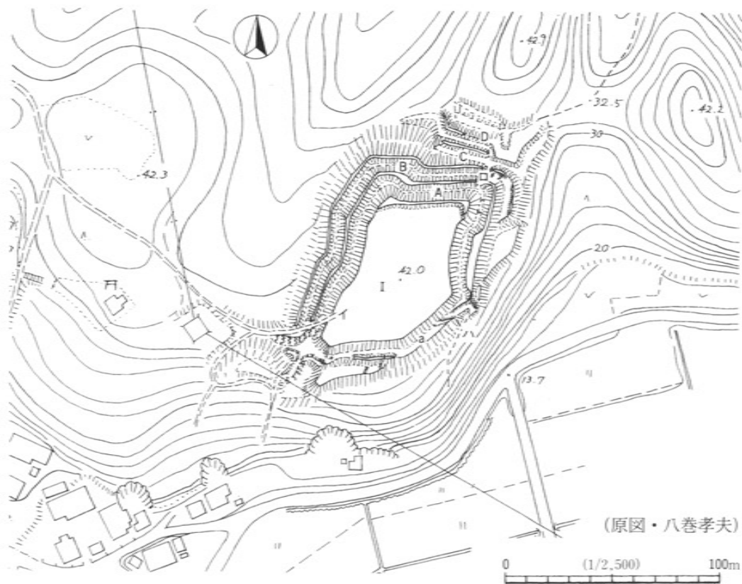
第68図 小見川町上小堀城跡(99)概念図 (最終Ⅲ期、城・城主クラスD) (『千葉県所在中近世城館跡詳細分布調査報告書 I』より)
