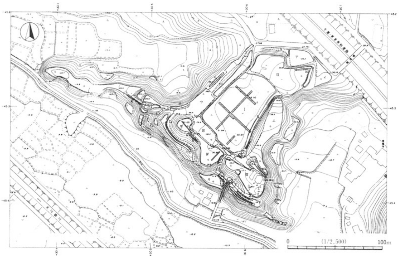
第47図 千葉市城山城跡(62)測量図 (最終Ⅲ期、城・城主クラスD) 〔千葉県中近世城跡研究調査報告書 第9集〕より
