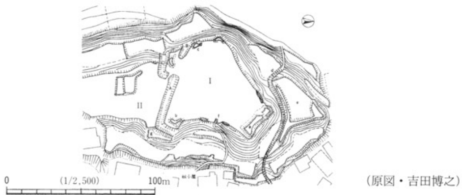
第60図 神崎町武田城跡(74)概念図 (最終Ⅲ期、城・城主クラスD) 〔千葉県所在中近世城館跡詳細分布調査報告書 I〕より
